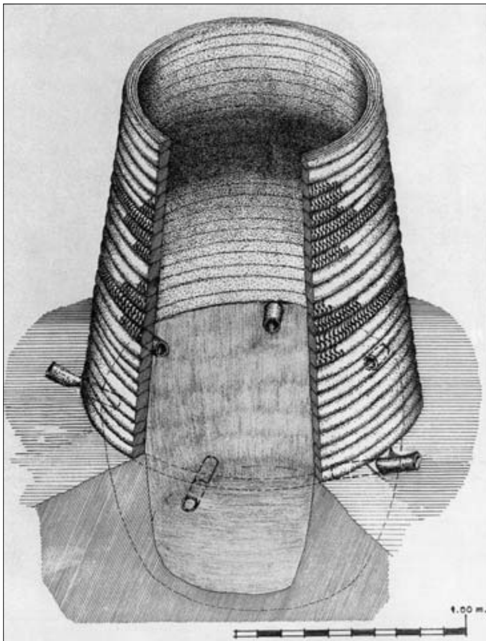
6.5. Exemple de reconstitution d'un fourneau de l'âge du fer ancien au Rwanda: Nyaruhengeri 1. [Source: C. Van Grunderbeek, E. Roche, H. Doutrelepont et P. Craddock, Musée royal de l'Afrique centrale, Tervuren, Belgique.]
